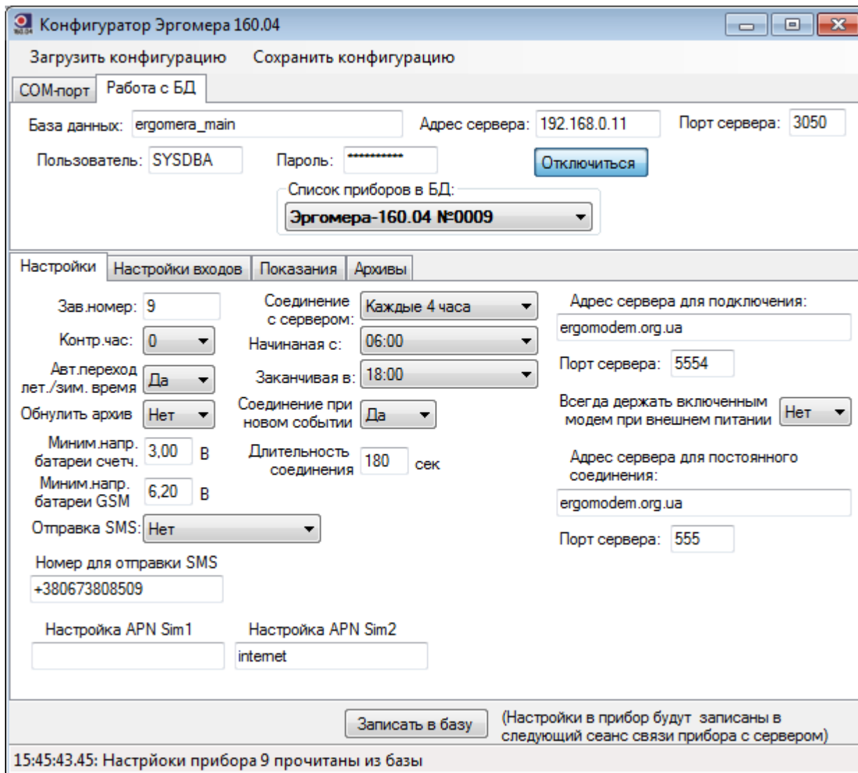
Рис.3 Вкладка «Работа с БД».
