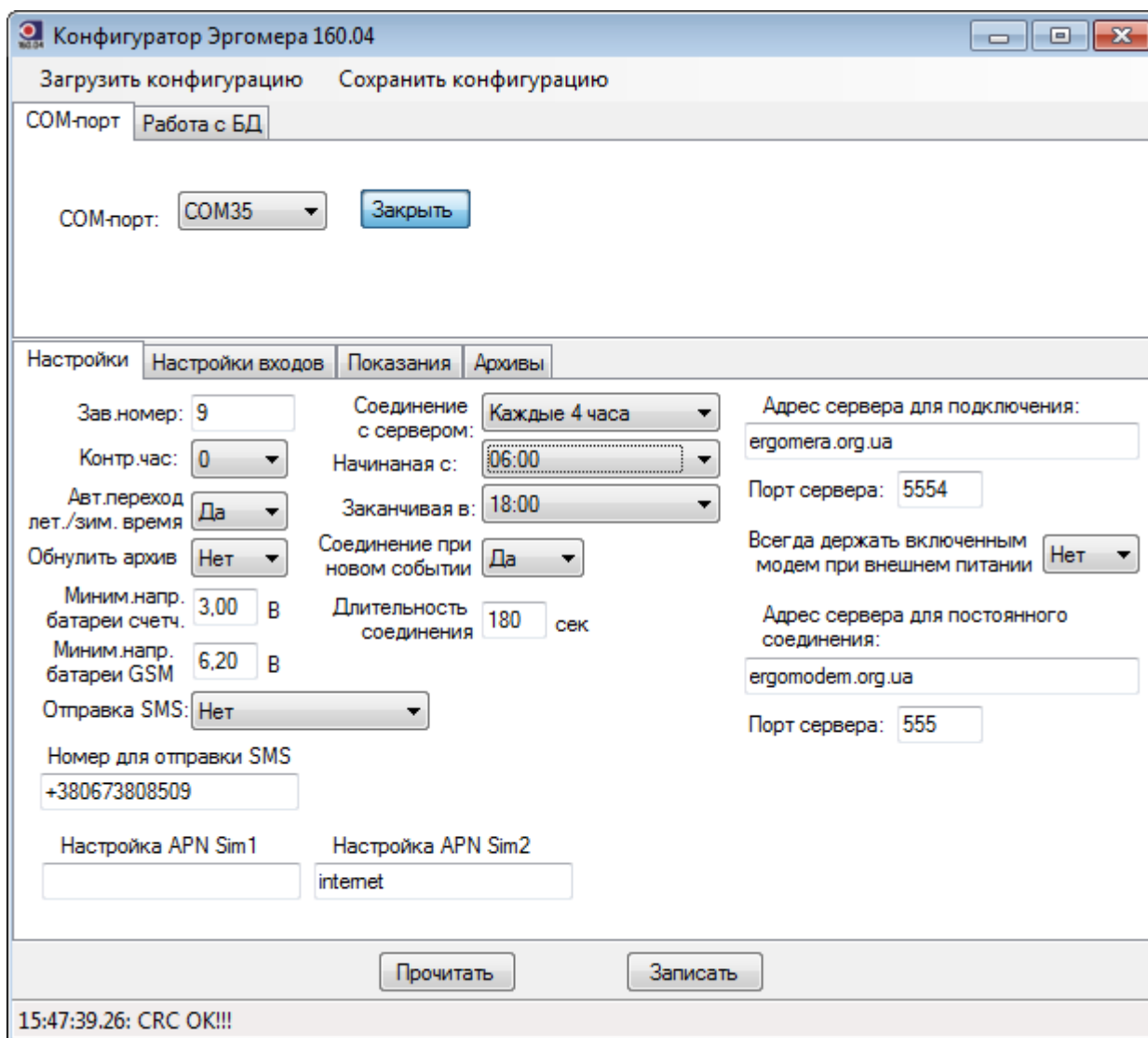
Рис.2 Вкладка «COM-порт».
