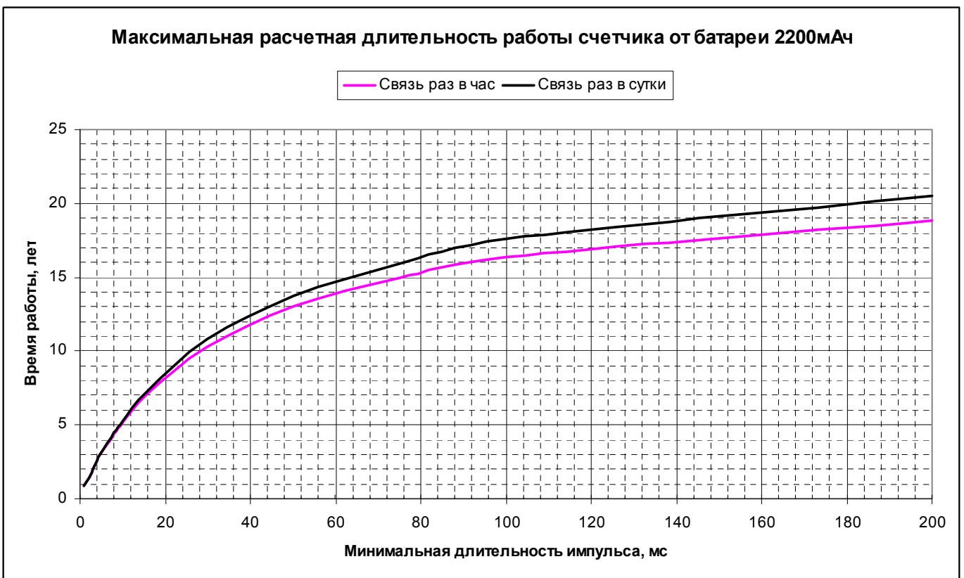
Рис. 2. Зависимость продолжительности работы батареи счетчика от минимальной длительности импульса и частоты связи с сервером для диапазона 1...200мс.
