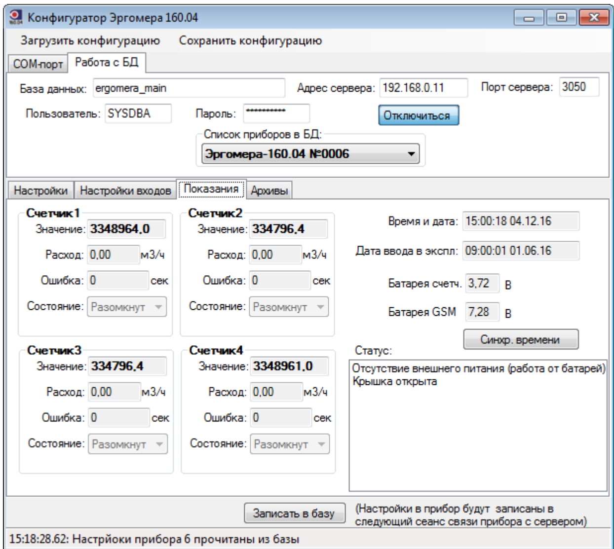
Рис.4 Вкладка «Показания».
